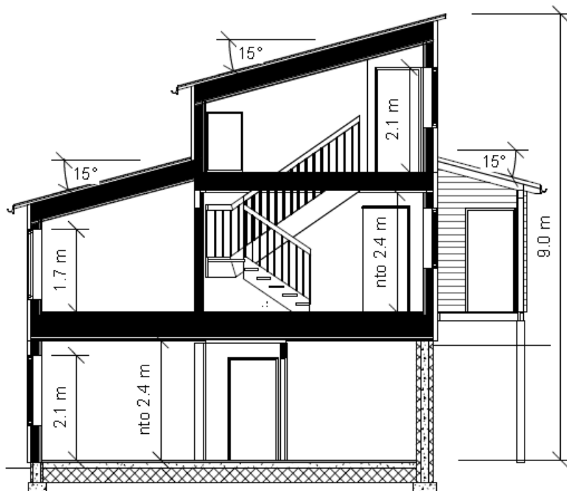
SNITT A-A
